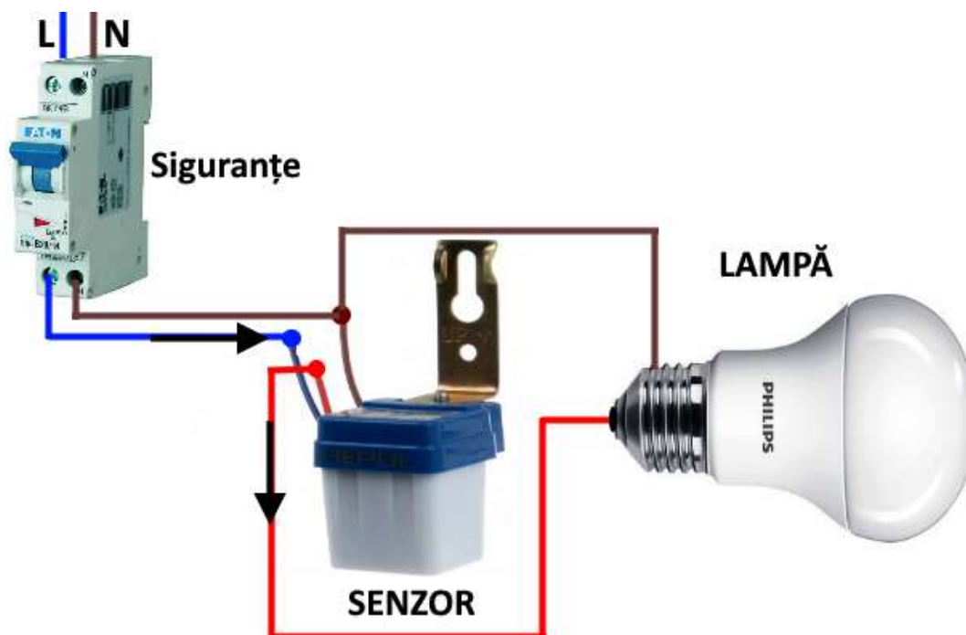
Figura 3.28 Conectare senzor de lumină crepuscular.
