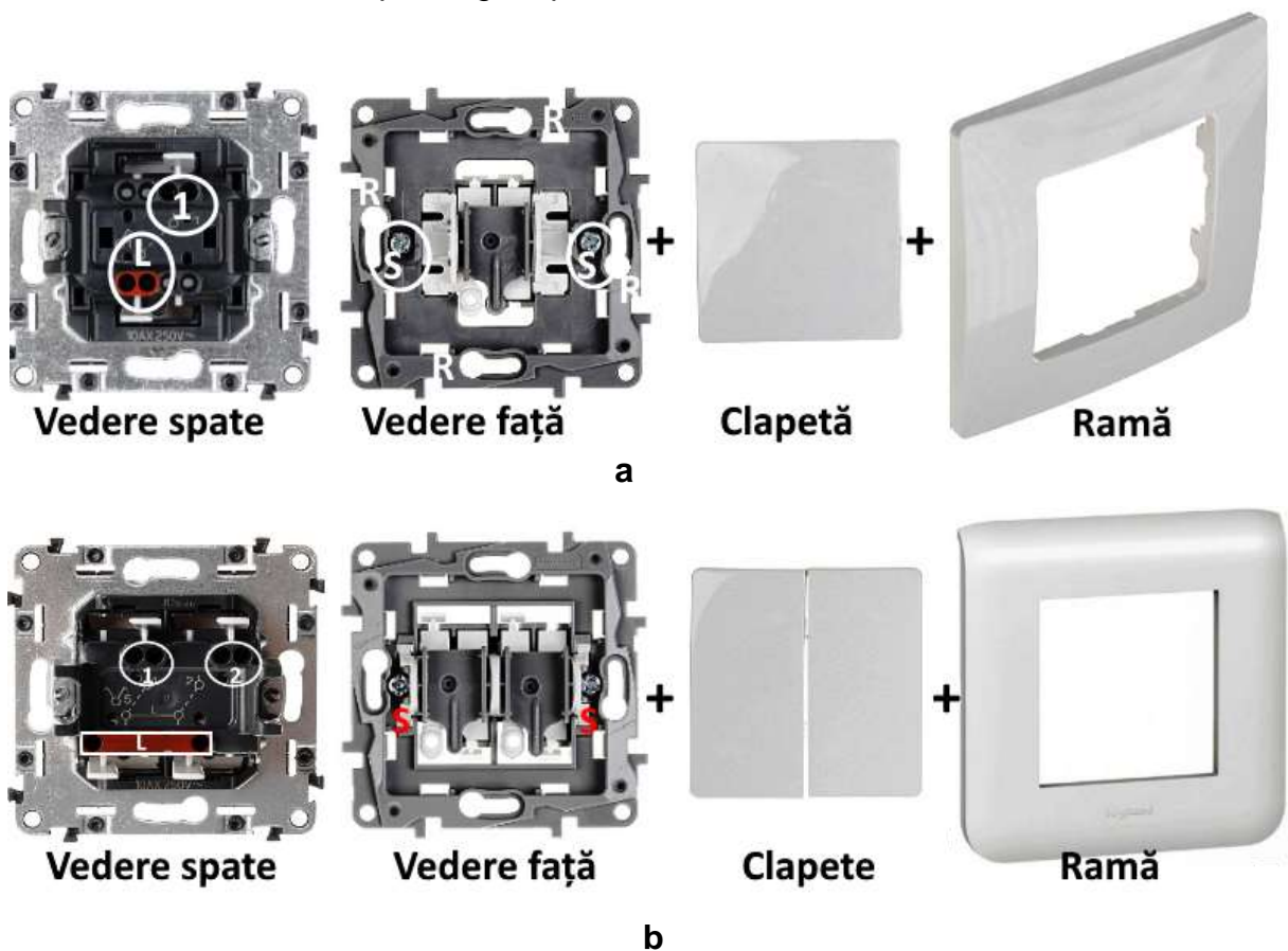
Figura 3.18 Montare întrerupător: a – simplu ; b – dublu
