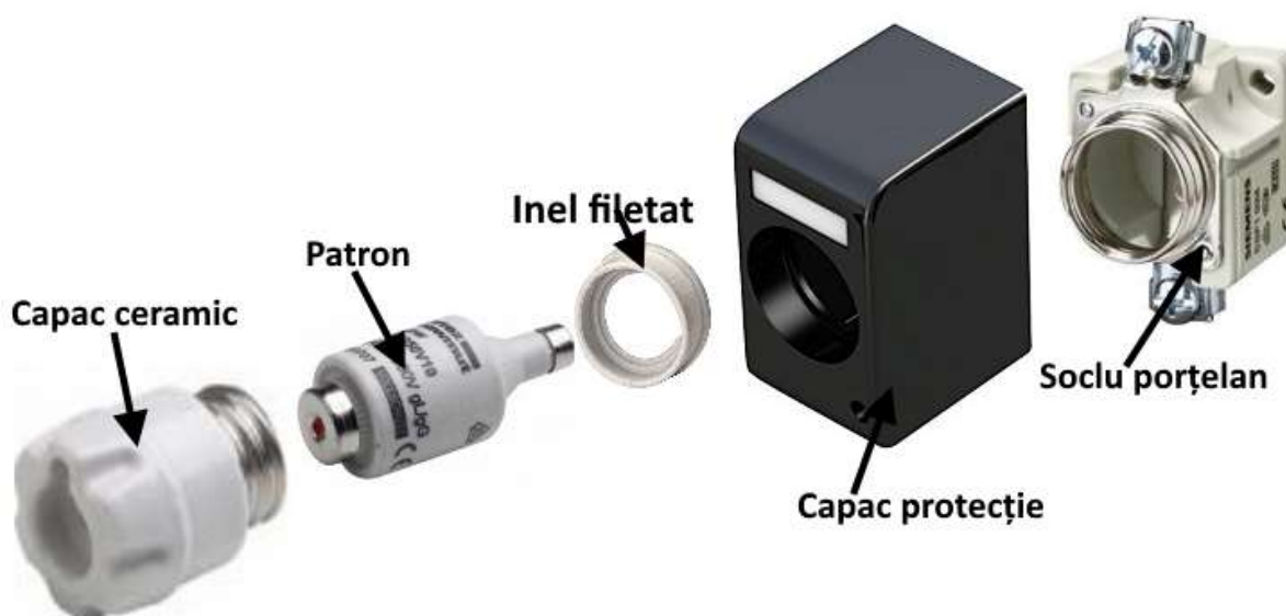
Figura 3.2 Elemente constructive siguranță fuzibilă cu filet
