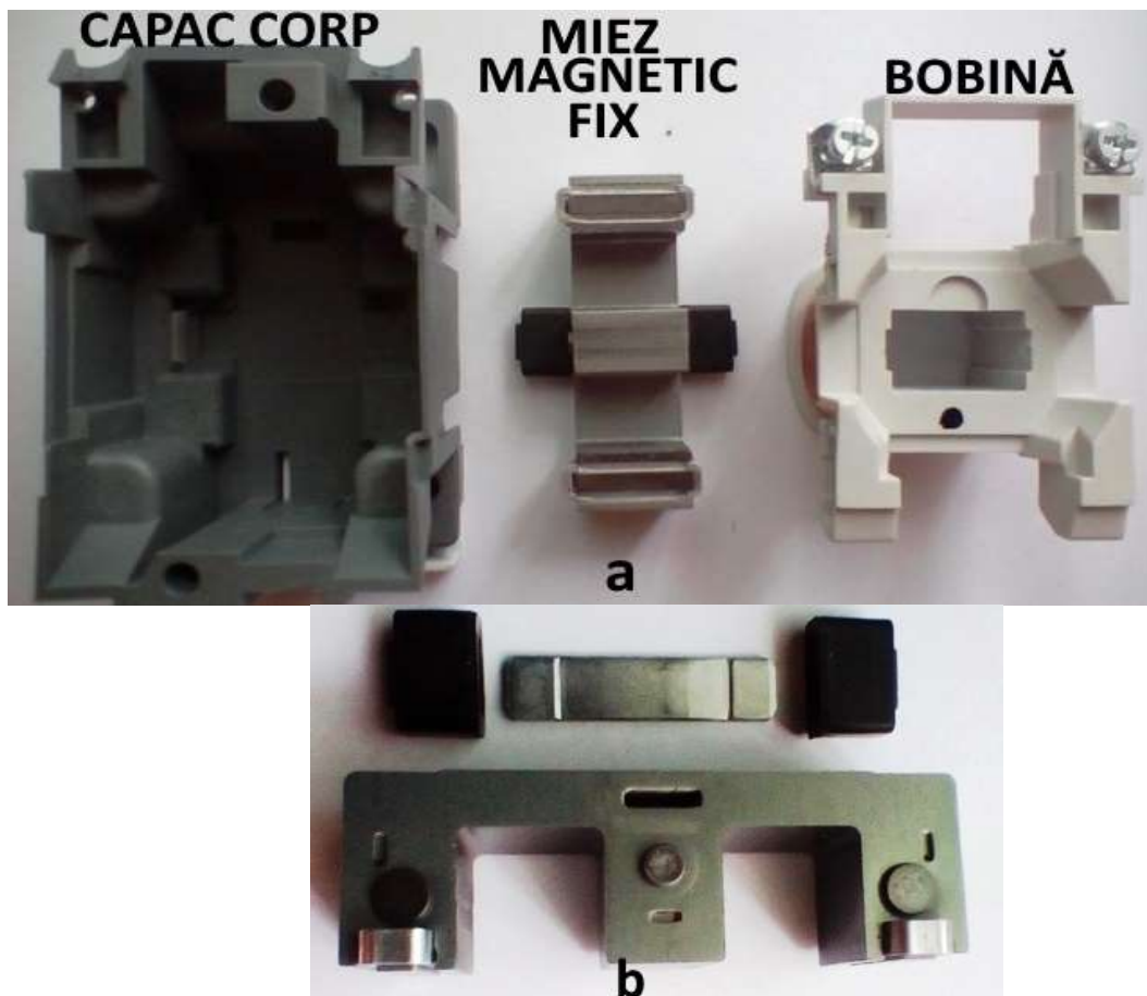
Figura 3.39 Demontare bobină și miez magnetic fix.
